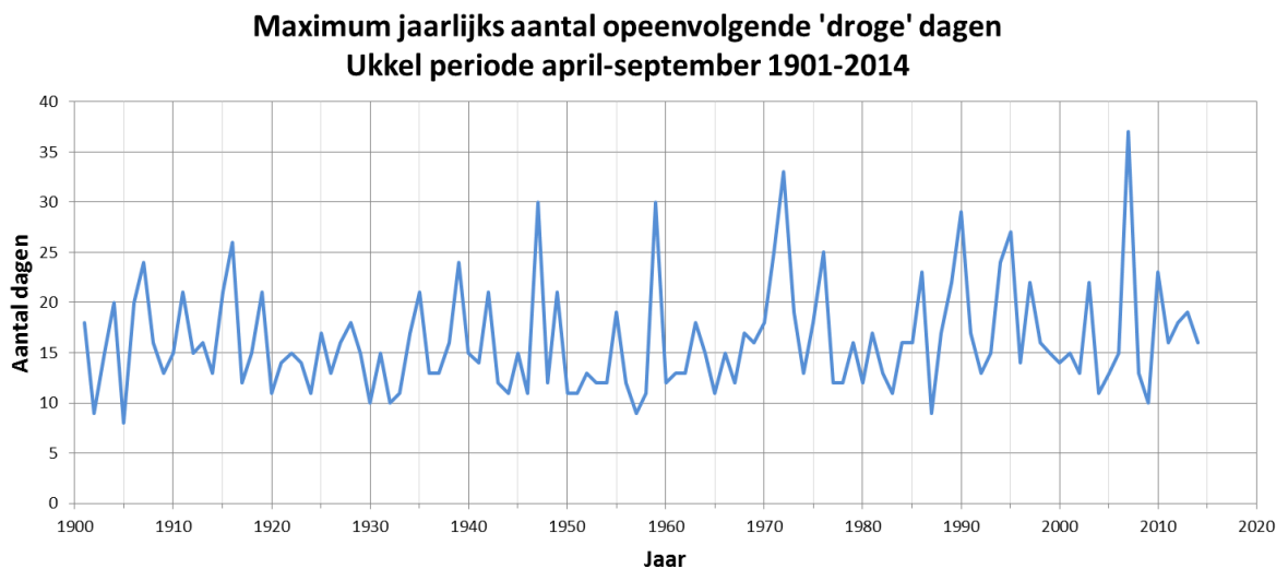
Figuur 1.23. Duur (in dagen) van de langste periode zonder significante neerslag (dagelijkse hoeveelheden kleiner dan 0,5 mm) gedurende de zes warmste maanden van het jaar te Ussel tijdens de periode 1901-2014.
