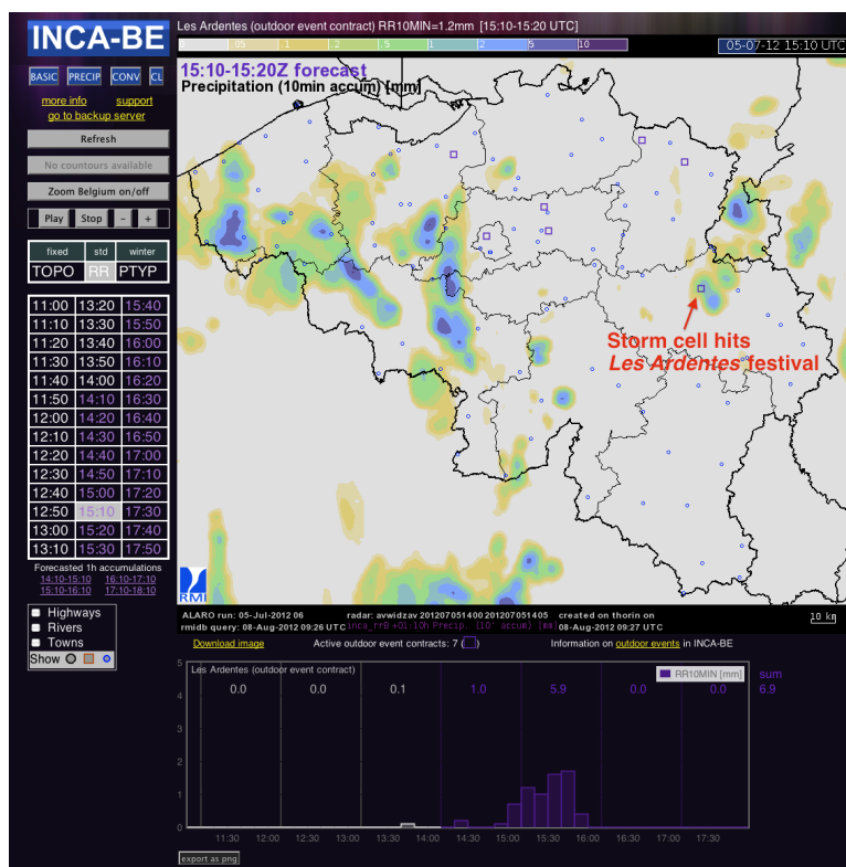
Figuur 4.11. Vooruitzichten voor de neerslag in het land tussen 15.10u en 15.20u UTC door het voorspellingssysteem van het KMI op zeer korte termijn, (INCA-BE), voor de onweerschtige periode van 5 juli 2012 (de kaart werd gemaakt om 14u UTC). Voor het terrein van het festival “Les Ardennes”, dat die dag in Luik doorging, toont het onderste deel van de afbeelding met intervallen van 10 minuten, ook de regenval (in mm) gemeten vóór 14u en de voorspelling tot 18u.
