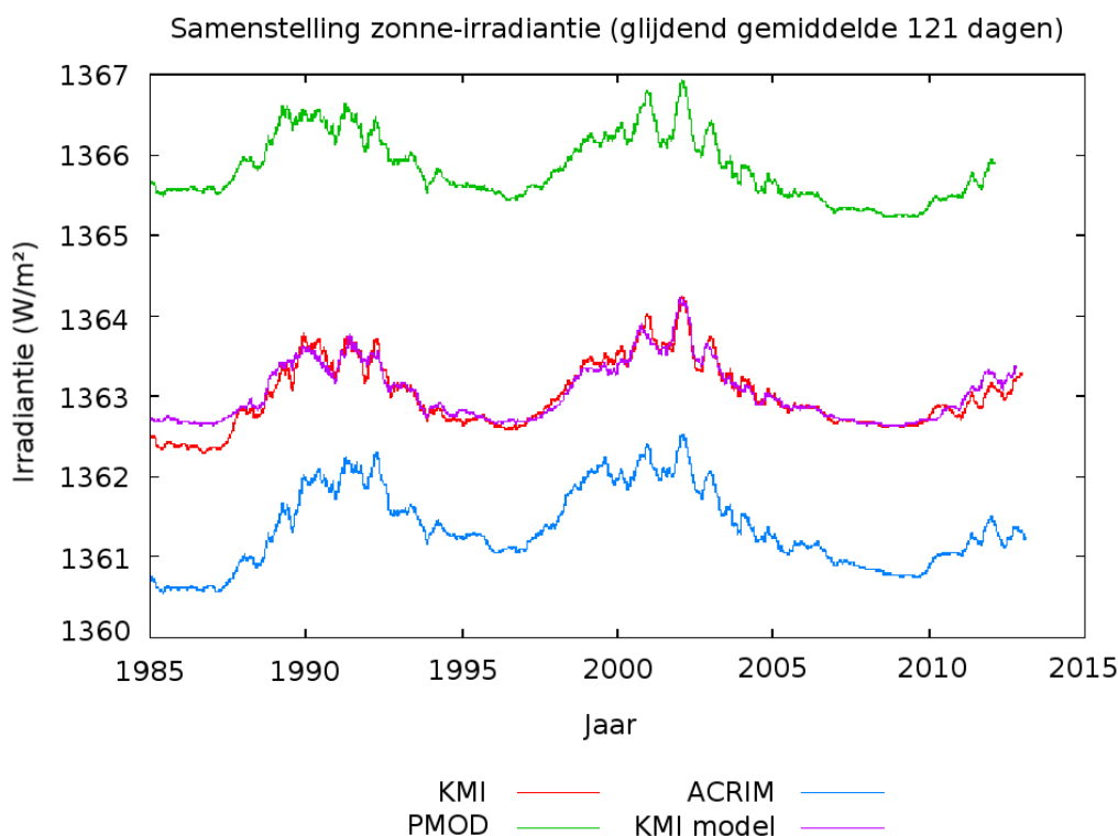
Figuur 2.1. Samenstelling van de metingen van de variaties van de totale zonnestraling (in \text{W/m}^2 voor de laatste twee elf-jarlijkse zonnecycli (cyclus 22, 23 en de start van cyclus 24)) door de drie internationale groepen KMI, PMOD en ACRIM. Het KMI-model is een regressiemodel dat gefit werd op de KMI-samenstelling van de metingen.
