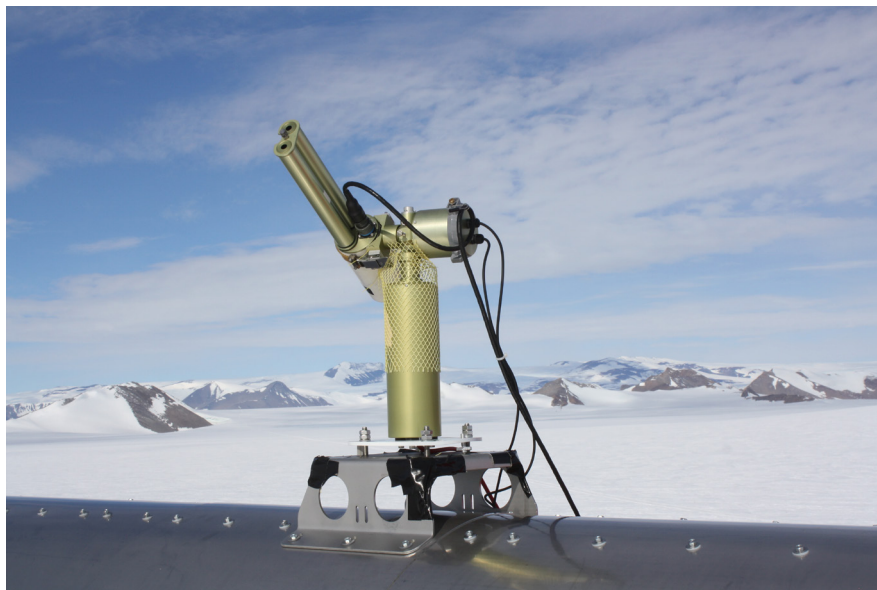
Figuur 2.17. Zonnefotometer gemonteerd op het dak van het Prinses Elisabeth Station, met uitzicht naar het zuidoosten. Deze fotometer meet op verschillende golflengten de demping van het zonlicht door atmosferische aerosolen.
