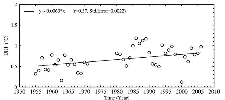
Figuur 4.3. De stadseffect op de gemiddelde minimum- en maximumtemperaturen voor de zomer tussen 1955 en 2006. Het stadseffect wordt geschat door het verschil tussen de temperaturen geregistreerd in het meetpunt in Ukkel en het landelijke meetpunt van Brussegem.
