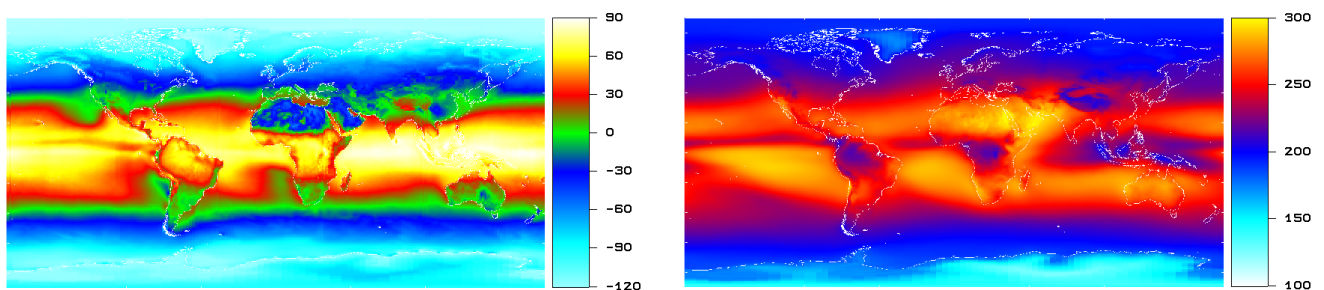
Figuur 2.6. 10 jaarlijkse CERES-klimatologie van de netto inkomende straling (links) en de uitgezonden thermische straling (rechts). De kleurschalen duiden energiestromen in W/m^2 aan.
