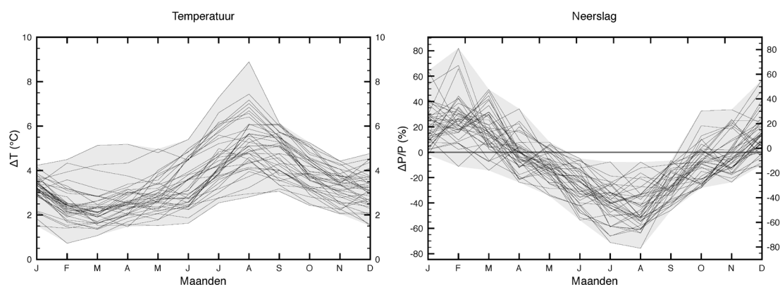
Figuur 4.6 Scenario's ontwikkeld op basis van het PRUDENCE-project voor veranderingen in de temperatuur ( \Delta T in ^{\circ}\text{C} , links) en relatieve veranderingen in neerslag (in \Delta P/P in %, rechts). Deze projecties zijn representatief voor België tijdens de periode van 2071 tot 2100. De curven stemmen overeen met de resultaten van 41 simulaties verkregen uit tien verschillende regionale klimaatmodellen en uitstootscenario's SRES A2 en B2.
