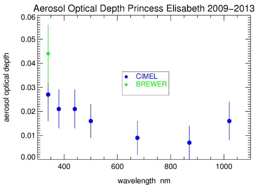
Figuur 2.18. Deze grafiek toont de gemiddelden (met foutenmarge) van het ultraviolet (340 nm) tot het dichtste infrarood (1020 nm) voor het 'Aerosol Optical Depth' (AOD, demping van zonlicht door de aerosolen) gedetecteerd door de zonnefotometer op verschillende golflengten (blauwe stippen). De groene stip wordt verkregen uit de gegevens van een Brewer spectrofotometer die ook op het dak van het station staat. De gemiddelden werden getrokken uit de gegevens gemeten tijdens elke zuidelijke zomer (december-februari) tussen 2009 en 2013.
