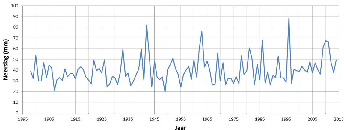
Figuur 1.17. Jaarlijkse maximale neerslaghoeveelheid gevallen in 24 uur (in mm) in Ukkel tijdens de periode 1898-2014.
