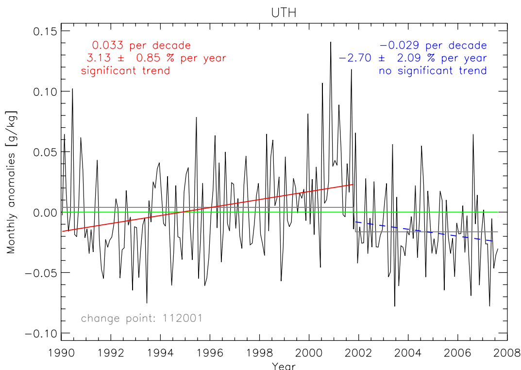
Figuur 2.14. Tijdreeks van de maandelijkse anomalieën van de hoeveelheid waterdamp in de bovenste troposfeerlagen in Ukel, uitgedrukt in g/kg. Een maandelijkse anomalie wordt verkregen door elke maand het langetermijnmaandgemiddelde af te trekken van het maandgemiddelde. Deze techniek heeft het voordeel dat de seizoencyclus verdwijnt uit een tijdreeks. De sterke afname van de hoeveelheid waterdamp in de herfst van 2001 is duidelijk zichtbaar.
