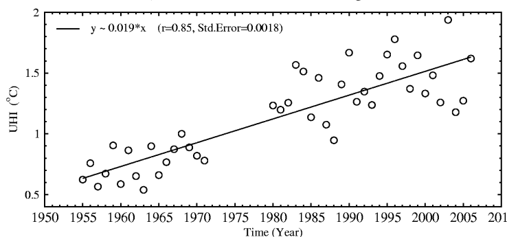
Figuur 4.3. De stadseffect op de gemiddelde minimum- en maximumtemperaturen voor de zomer tussen 1955 en 2006. Het stadseffect wordt geschat door het verschil tussen de temperaturen geregistreerd in het meetpunt in Ukkel en het landelijke meetpunt van Brussegem.
