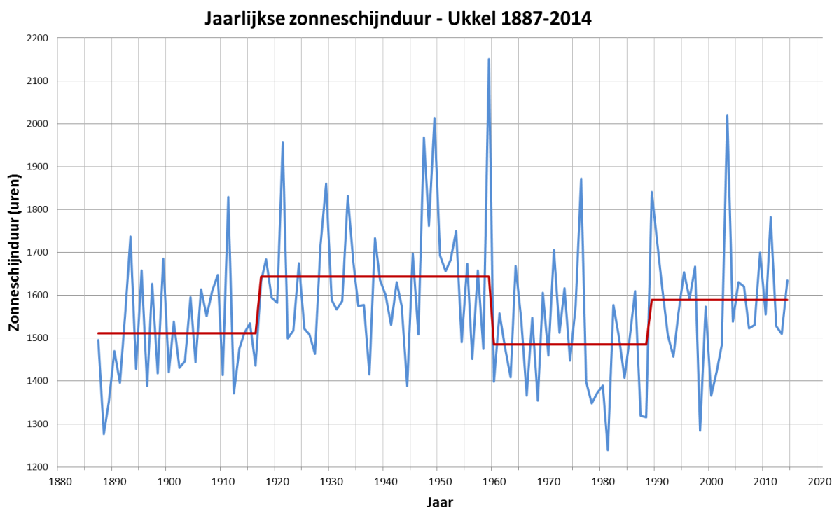
Figuur 1.27. Jaarlijkse zonneschijnduur (in uren) in Ukkel tijdens de periode 1887-2014.
