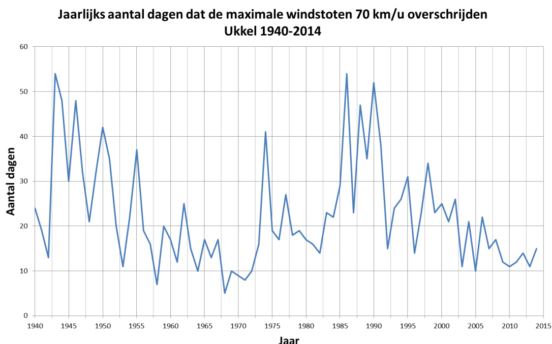
Figuur 1.26. Jaarlijks aantal stormdagen (maximale windstoot hoger dan 70 km/u) te Ukkel tijdens de periode 1940-2014.
