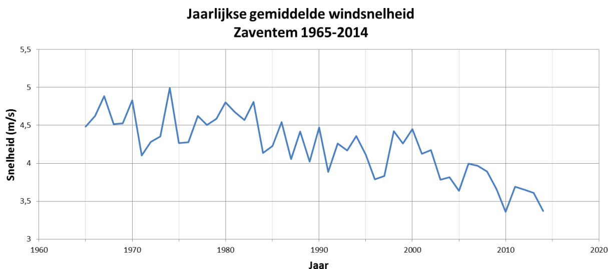
Figuur 1.25. Jaarlijkse gemiddelde windsnelheid, te Zaventem tijdens de periode 1965-2014 (in m/s).
