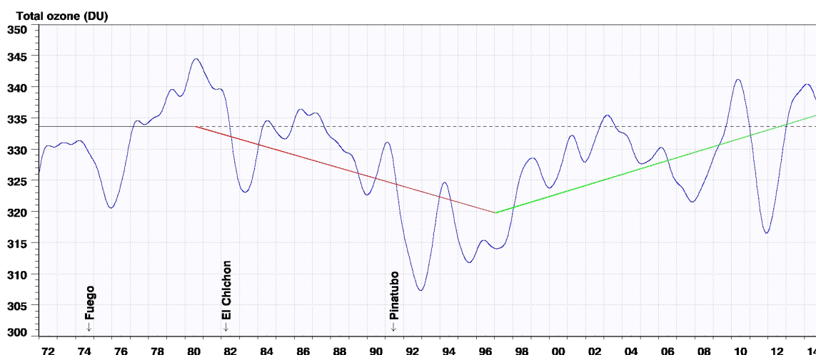
Figuur 2.12. Dikte van de ozonlaag (in DE) boven Ukkel met stapsgewijze trendberekening (1972-2014).
