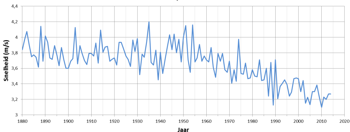
Figuur 1.24. Jaarlijkse gemiddelde windsnelheid in Sint-Joost-ten-Node/Ukkel tijdens de periode 1880-2014 (in m/s).
